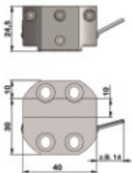
Bild 1 R + L + überkopf einsetzbar Useable r., l. + overhead
