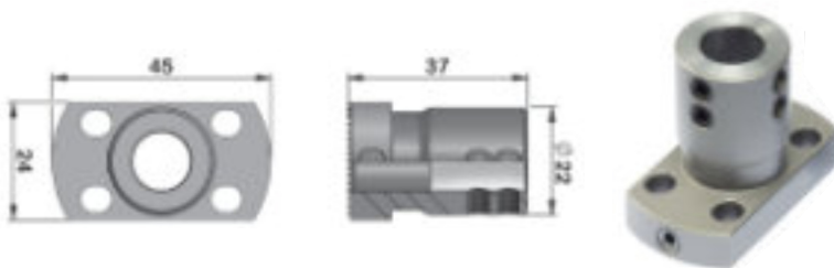
Bild 1: Halter - holder
