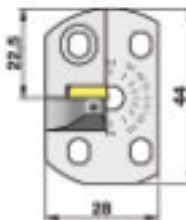
Ausführung rechts (Version right)
