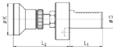
Ausführung mit VDI-Schaft
